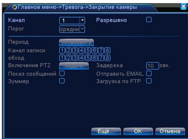
Рисунок 4.6 Закрытие камеры
