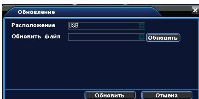
Рисунок 4.32 Обновление
