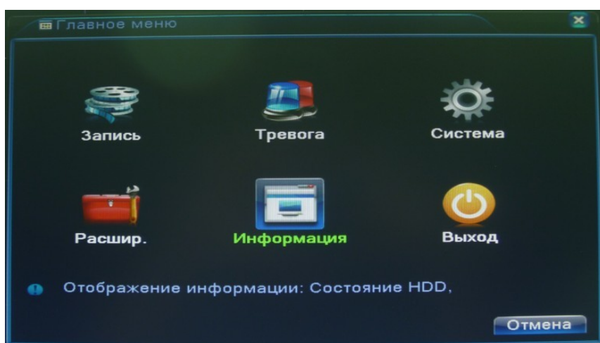
Рисунок 3.3 Главное меню
