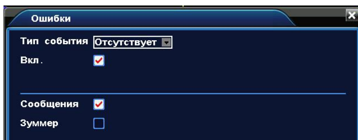
Рисунок 4.9 Ошибки
