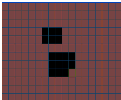
Рисунок 4.3 Зона
