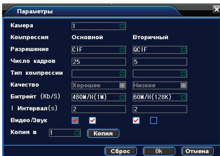
Рисунок 4.11 Установка кодирования
