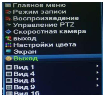
Рисунок 3.2 Контекстное меню
