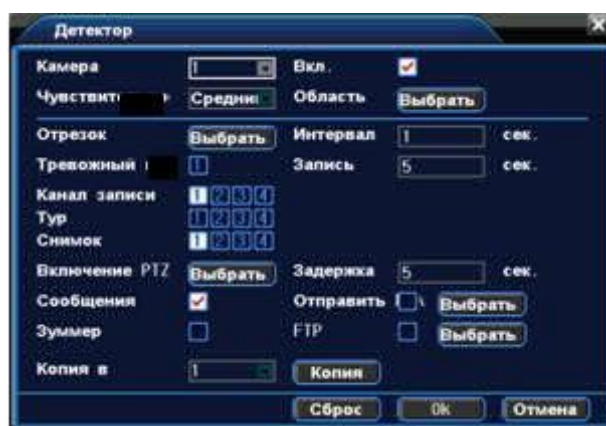
Рисунок 4.2 Детектор движения
