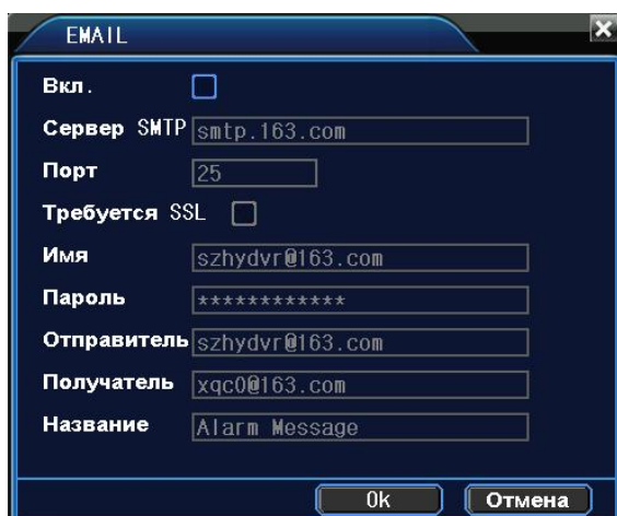
Рисунок 4.16 EMAIL
