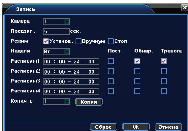
Рисунок 4.1 Конфигурация записи
