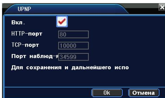
Рисунок 4.20 UPNP
