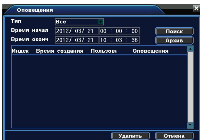
Рисунок 4.36 Журнал
