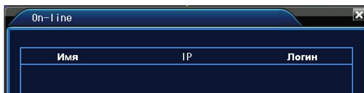
Рисунок 4.29 Пользователи сети
