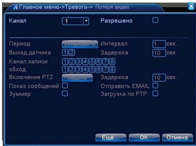
Рисунок 4.7 Потеря видеосигнала
