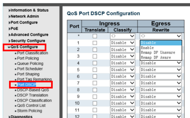
Рисунок 6-7 Экран DSCP Конфигурации порта
