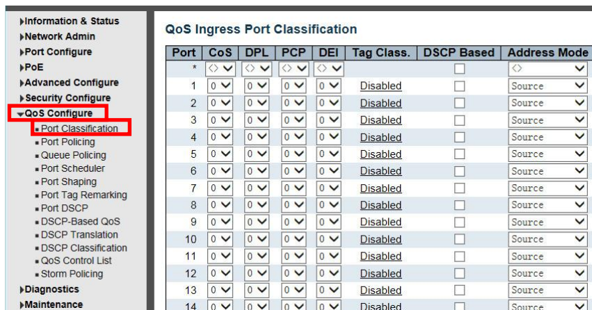
Рисунок 6-1 Экран конфигурации классификации портов
