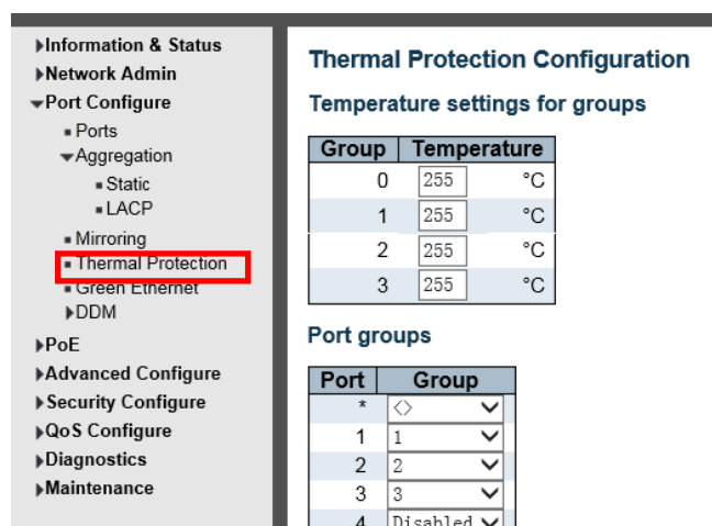
Рисунок 3-4. Экран настройки термозащиты
