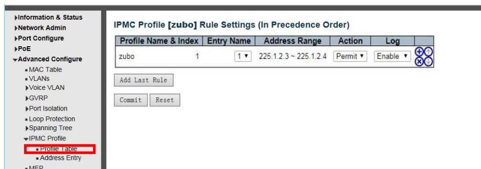
Рисунок 5-5-2 Экран настройки правила фильтрации для определенного профиля IPMC.
