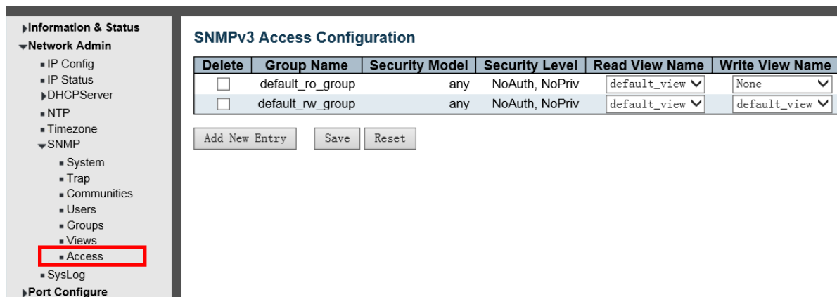
Рисунок 2-6-7 Настройка доступа SNMPv3
