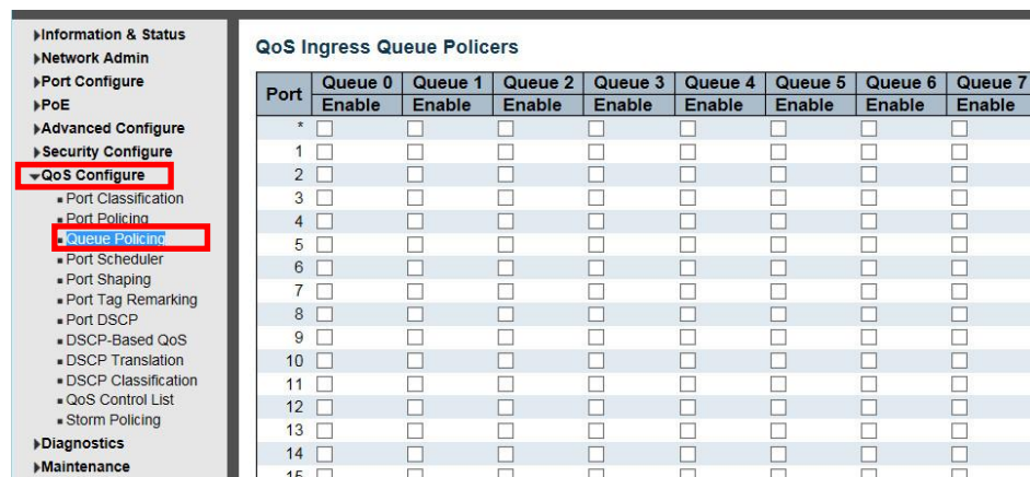
Рисунок 6-3 Экран конфигурации ограничителя очереди входящего трафика QoS
